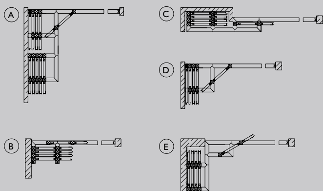
Voorbeelden 90° opstellingen:
