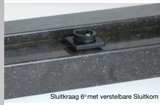
Onderdorpel Belgisch hardsteen
